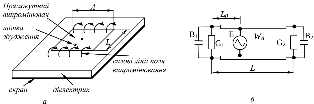
Рис. 2. Мікросмужкова антена (а) та схема її заміщення (б)
