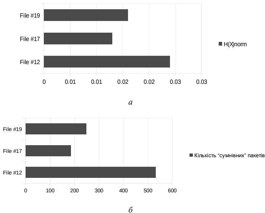
Рис. 2. Порівняння показників нормалізованої ентропії (а) і кількості “сумнівних” пакетів (повторної передачі, деформованих тощо) (б)
