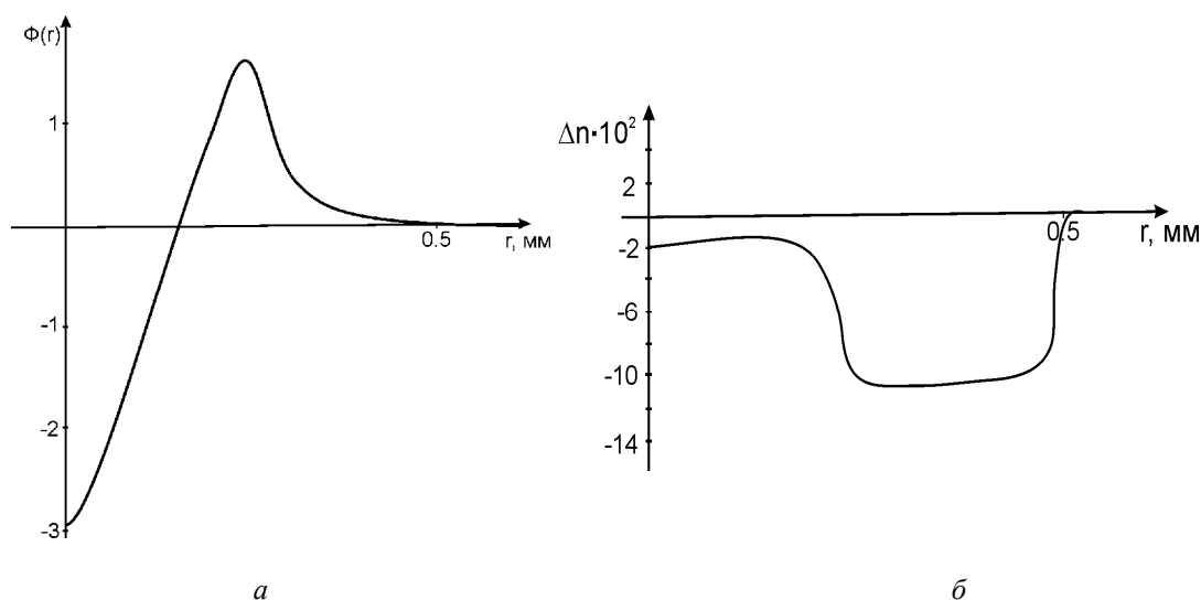
Рис. 5. Розшифрування інтерферограми: а – функція зміни оптичної довжини шляху променя в об'єкті; б – розподіл показника заломлення в поперечному перерізі волокна відносно показника заломлення іммерсійної рідини ( n=1,511 )
