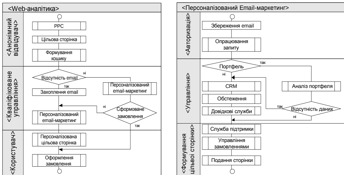
Рис. 7. Схема аналізу контенту відвідувачів (а) та інформаційного ресурсу (б)
