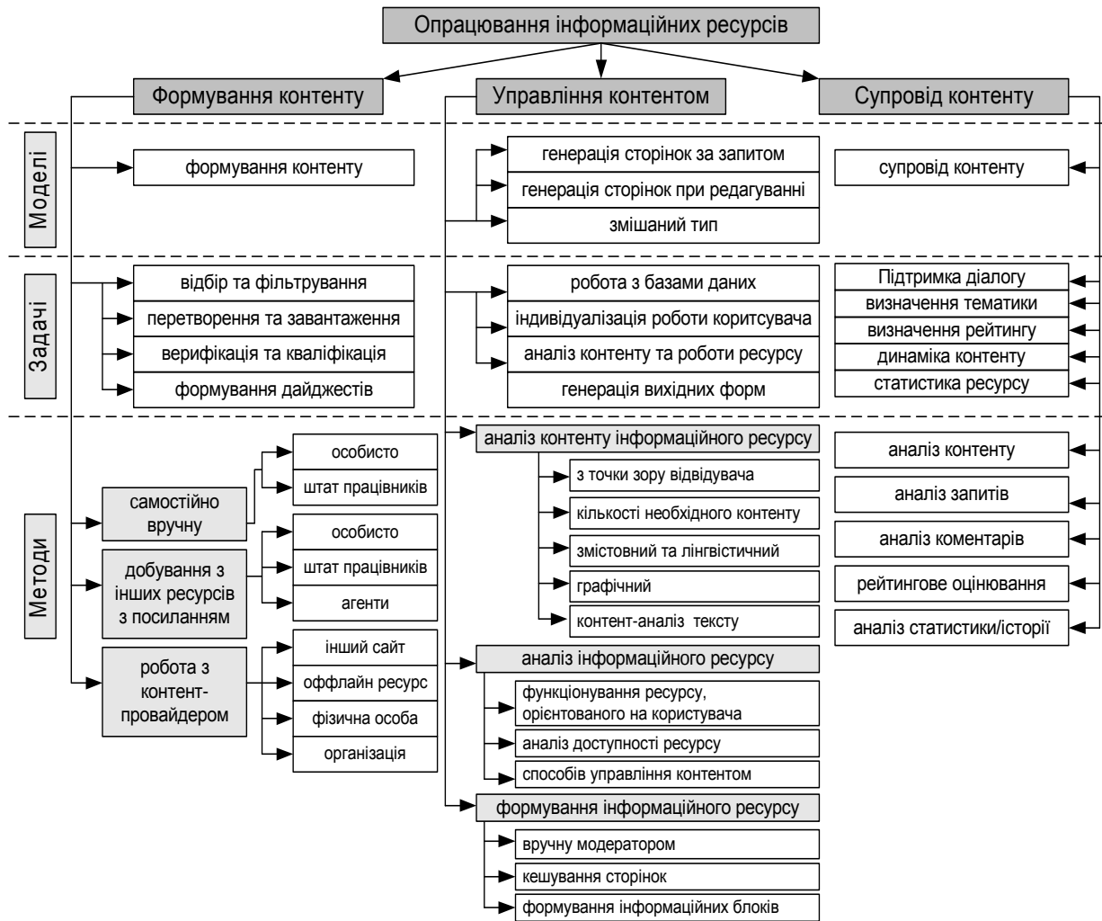
Рис. 12. Особливості процесу опрацювання інформаційних ресурсів СЕКК
