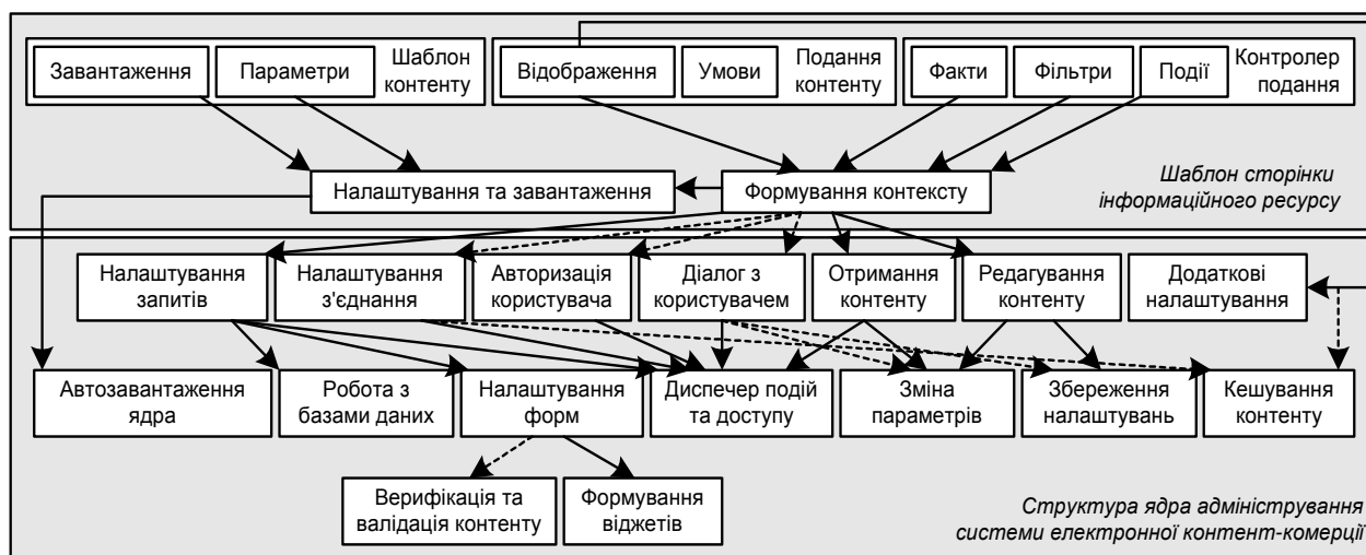
Рис. 4. Діаграма структури системи електронної контент-комерції
