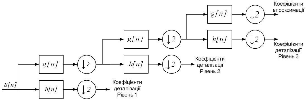
Рис.2. Трьохрівневий банк фільтрів
