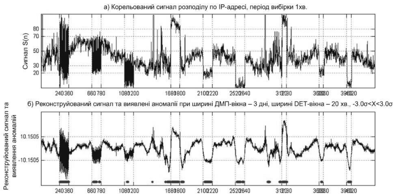
Рис.5. Розподіл при наявності атаки.
