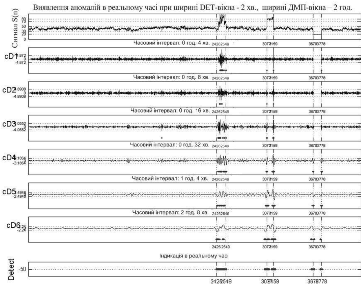
Рис.6 Результати виявлення атак в реальному часі з використанням ДМП.
