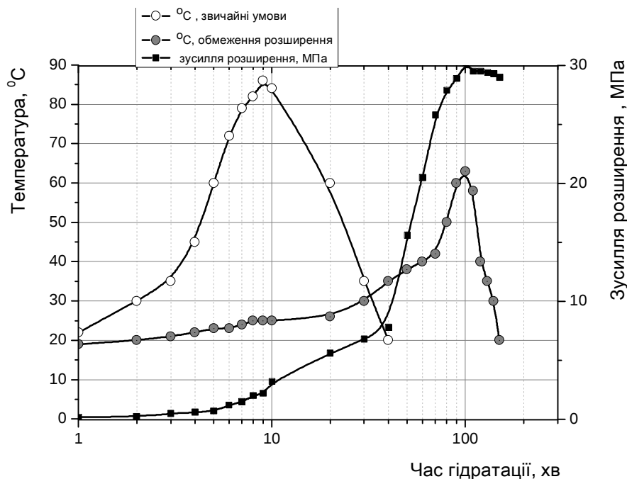
Рис. 1. Вплив умов гідратації СаО на кінетику зміни температури та зусилля розширення ( B/B = 1,0 )
