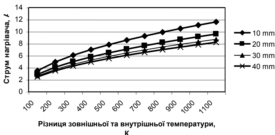
Рис. 4. Залежність необхідного струму нагрівача від товщини теплоізоляційного шару (мм)
