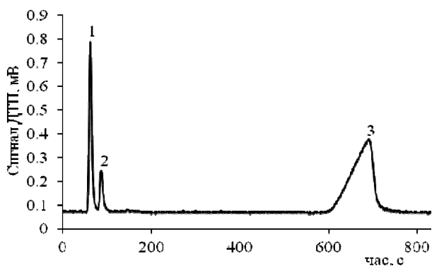
3 пік – ГЕТМЦГК
