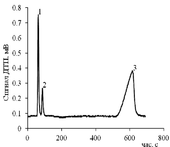
3 пік – АТМЦГК
