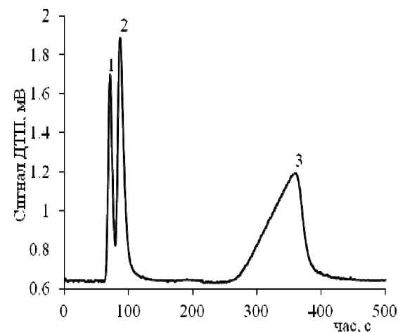
3 пік – МДМЦГК
