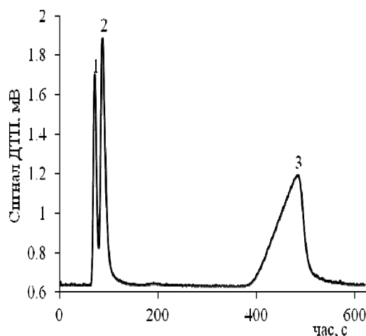
3 пік – МТМЦГК
