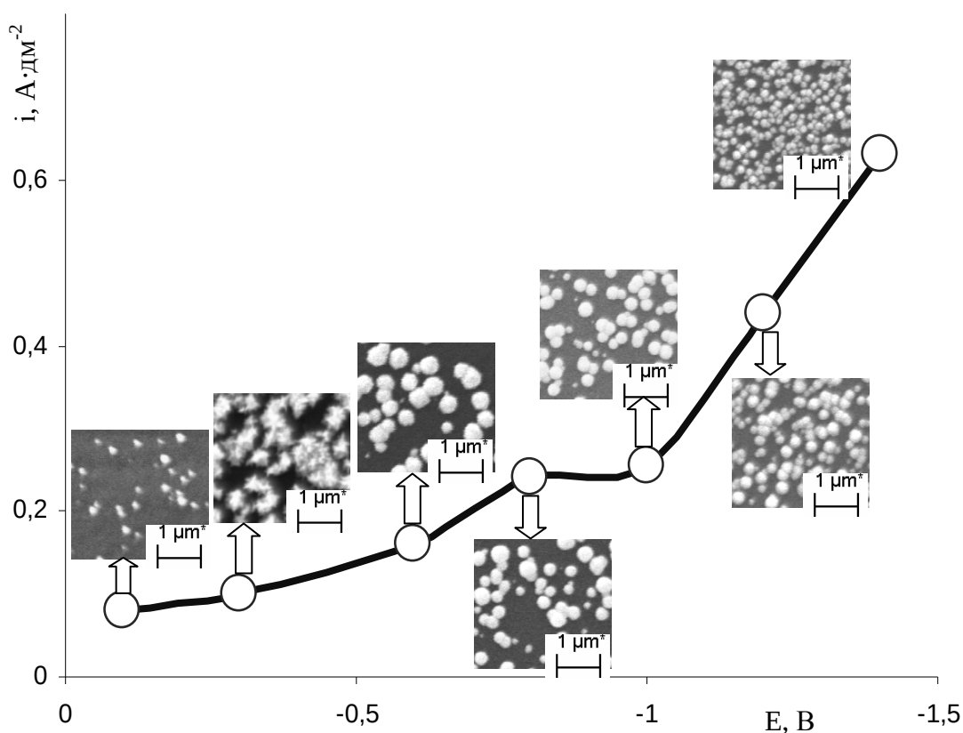
Рис. 2. Стилїзована крива морфології золота, нанесеного на склографіт із 0.004M \text{H[AuCl}_4\text{]} + 0.05\text{M Bu}_4\text{NClO}_4 у розчинах DMF за 35 °C залежно від катодного потенціалу за імпульсного режиму
