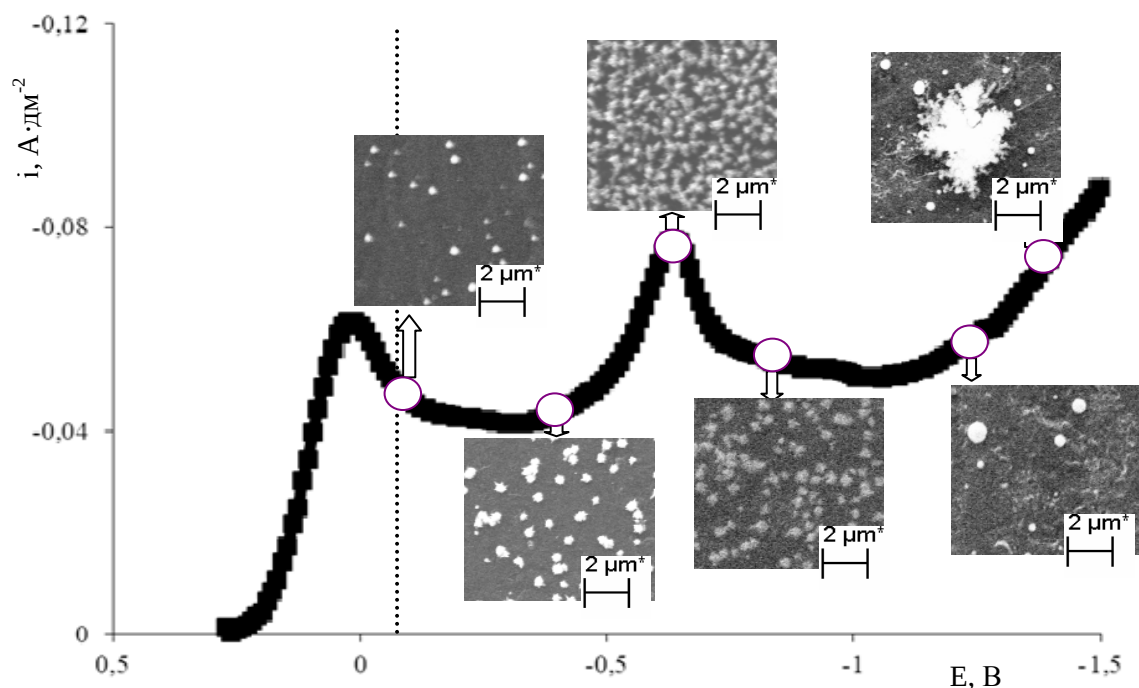
Рис. 1. Стилзована крива морфології золота, нанесеного на склографіт із 0.004 M \text{HAuCl}_4 + 0.05 M \text{Bu}_4\text{NClO}_4 у розчинах DMF за 35 °C залежно від катодного потенціалу
