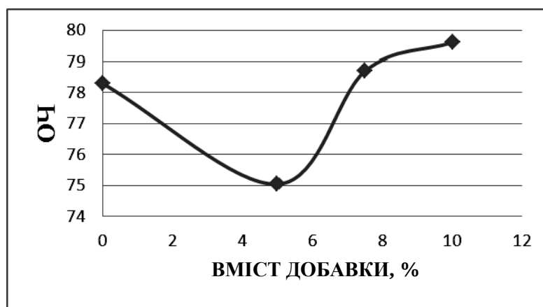
Рис. 1. Залежність ОЧ від конентрації СО (%) у бензині А-78
