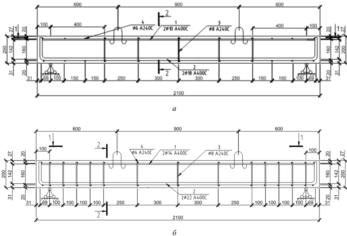
Рис. 6. Армування та розміри дослідних балки: а – балка без поперечного армування; б – балка з поперечним армуванням
