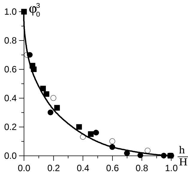
Рис. 3. Залежність \Phi_0^3 від безрозмірної довжини шару. Точки відповідають експериментальним даним у випадку екстрагування цільових компонентів, зокрема:
