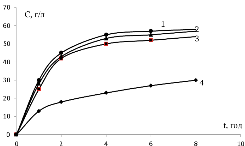
Рис. 4. Залежність c=f(t) екстрагування олії з насіння ріжжію d_{\text{сер}}=0,25 мм різними розчинниками за температури їх кипіння: 1 – хлористий метилен ( t_{\text{кип.}}=41^\circ\text{C} ); 2 – хлороформ ( t_{\text{кип.}}=67^\circ\text{C} ); 3 – н-гексан ( t_{\text{кип.}}=62^\circ\text{C} ); 4 – етанол ( t_{\text{кип.}}=78,3^\circ\text{C} )
