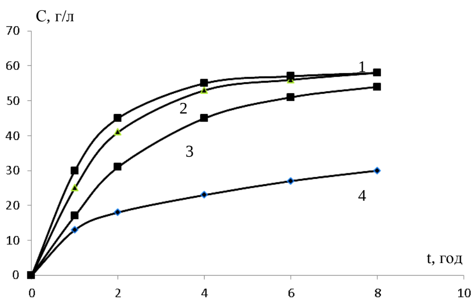
Рис. 5. Залежність c=f(t) екстрагування олії з насіння ріжю за температури 40^{\circ}\text{C} різними розчинниками: 1 – хлористий метилен; 2 – хлороформ; 3 – н-гексан; 4 – етанол
