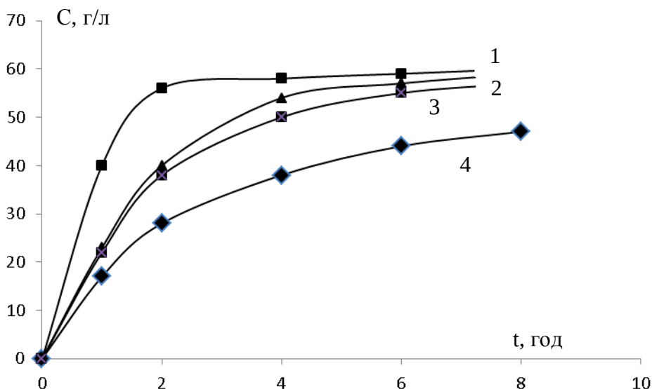
Рис. 2. Залежність c=f(t) екстрагування олії хлористим метиленом із подрібненого насіння ріжю за температури 40^\circ\text{C} : 1 – d_{\text{сер}}=0,16 мм; 2 – d_{\text{сер}}=0,25 мм; 3 – d_{\text{сер}}=0,35 мм; 4 – d_{\text{сер}}=0,5 мм
