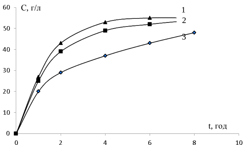
Рис. 3. Залежність c=f(t) екстрагування олії н-гексаном із насіння ріжю за d_{\text{сер}}=0,25 мм за різних температур: 1 – 60 °C; 2 – 40 °C; 3 – 20 °C
