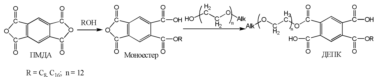
Рис. 1. Схема синтезу амфіфільних дієстерів піромелітової кислоти
