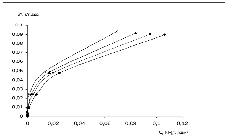
Рис. 1. Статична ємність ґрунтів щодо \text{NH}_4^+ : ◆ – пісок; ■ – чорнозем; ▲ – торф; x – глина
