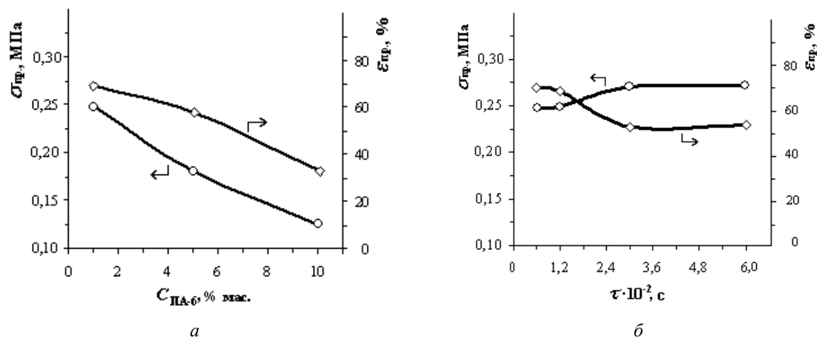
Рис. 1. Залежність міцності ( \sigma_{np} ) і видовження ( \epsilon_{np} ) у разі прориву тонкоплівкових композитів на основі рідкоструктурованих кополімерів ГЕМА:ПВП від концентрації ПА-6 ( C_{ПА-6} ) у модифікувальному розчині (а) і часу ( t_{yn.} ) упарювання розчинника (б): Розчинник: HCOOH:H_2O = 80:20 мас. %; T_{yn.} = 60^\circ C ; а- t_{yn.} = 0,6 \cdot 10^{-2} с; б- C_{ПА-6} = 1 % мас.
