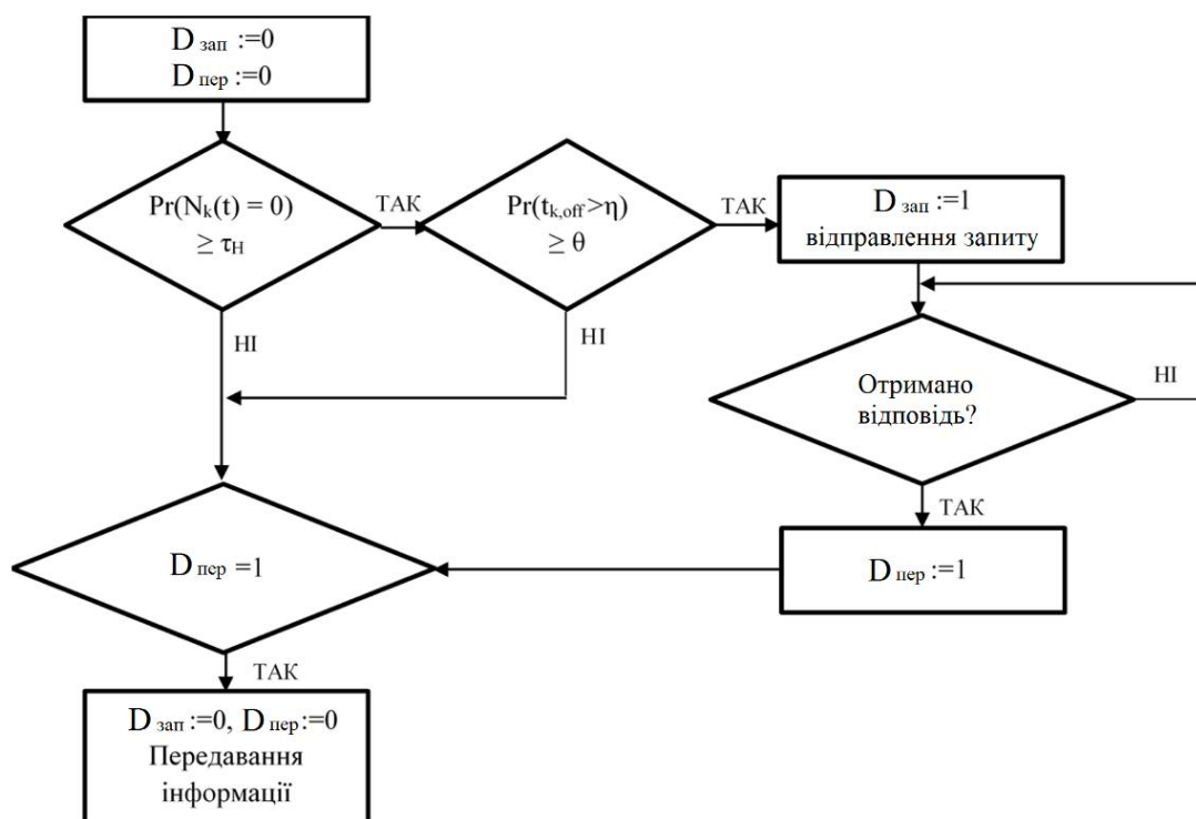
Рис. 3. Алгоритм початку нової передачі:
