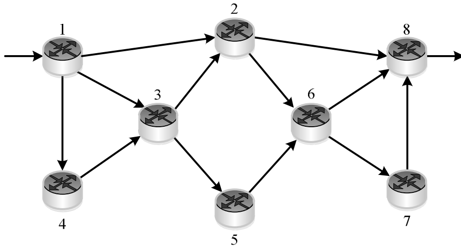
Рис. 3. Приклади шляхів, що перетинаються за вузлами
