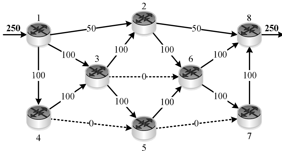
Рис. 5. Результат розрахунку множини шляхів з використанням умов (4) маршрутизації за шляхами, що перетинаються за вузлами, у разі обслуговуванні потоку інтенсивністю 250 1/с
