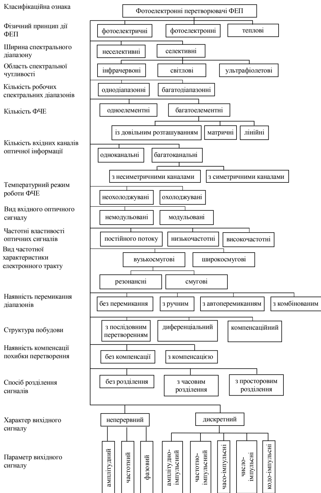
Рис. 2. Класифікація ФЕП, придатних для використання в СТOM
