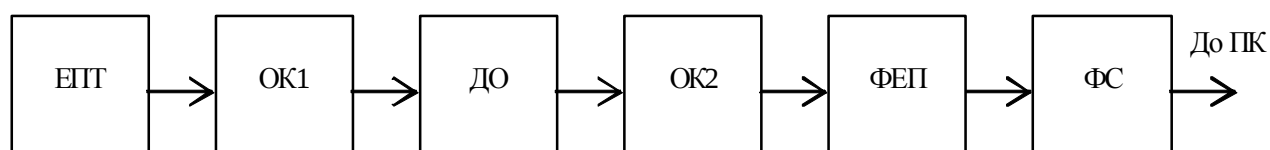
Рис. 1. Структурна схема СТОМ з погляду формування відеосигналу
