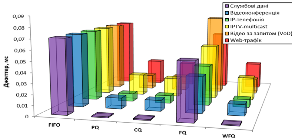
Рис. 7. Джитер для різних потоків при використанні відповідного алгоритму обслуговування
