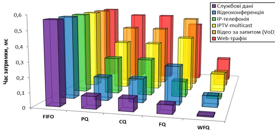
Рис. 6. Час затримки для різних потоків при використанні відповідного алгоритму обслуговування
