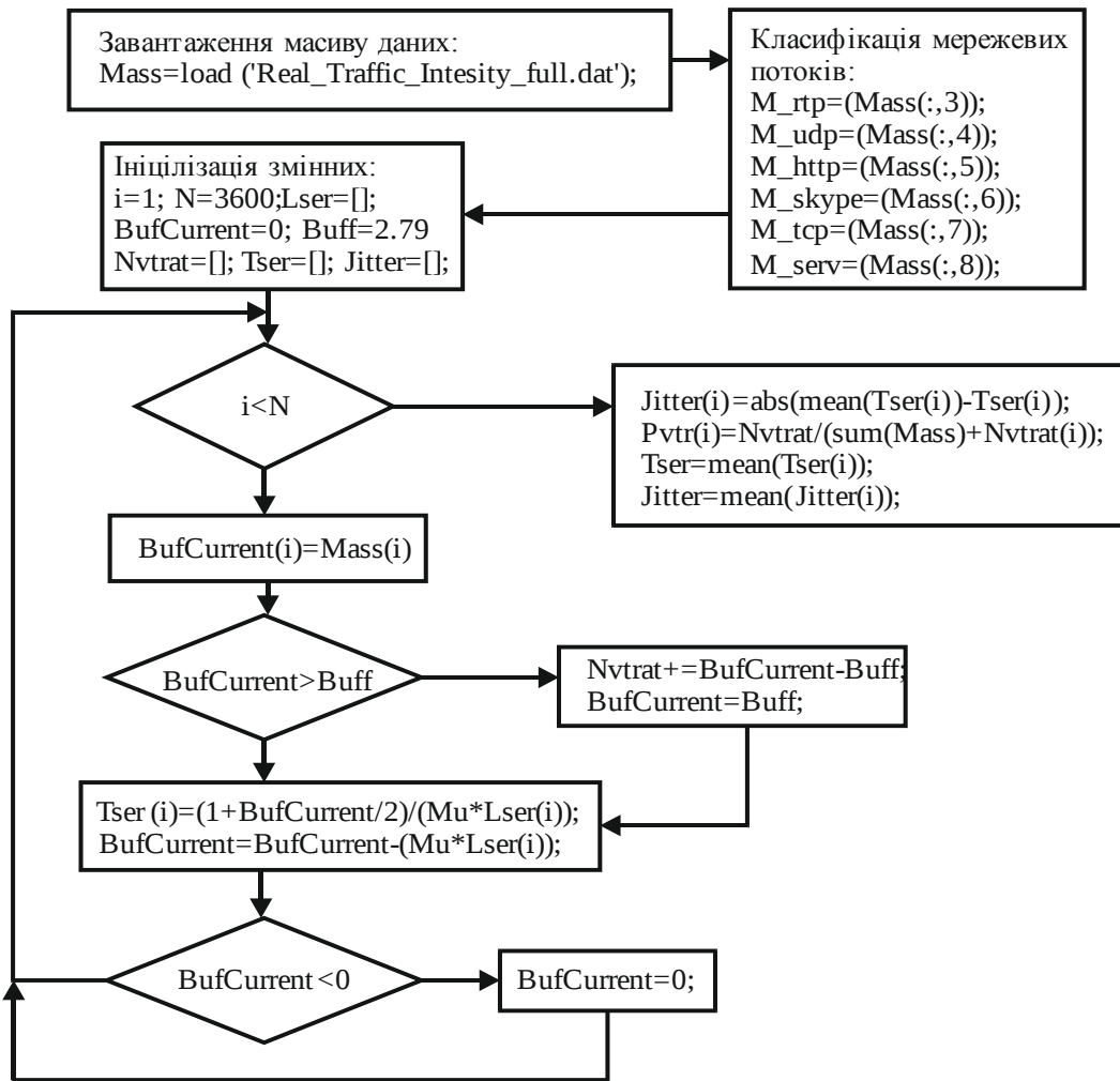
Рис. 4. Алгоритм роботи імітаційної моделі
