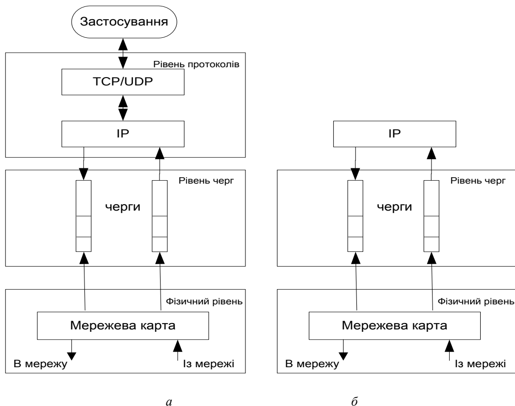
Рис. 2. Модель взаємодії мережевого стеку
