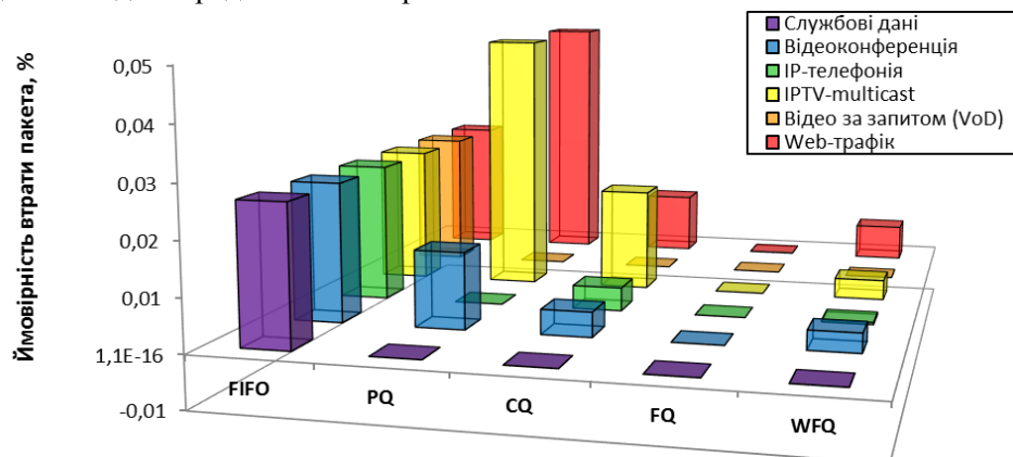
Рис. 5. Ймовірність втрати пакетів для різних потоків при використанні відповідного алгоритму обслуговування
