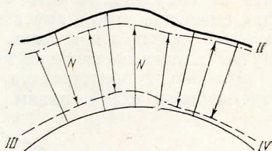
Рис. 1. Расположение геоидов (I, II, III) относительно сфероида (IV):
