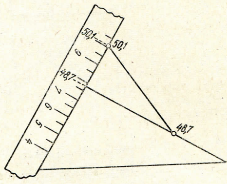
Рис. 4. Пример интерполирования горизонталей одной линейкой и угольником. Угольник движется вдоль линейки.
