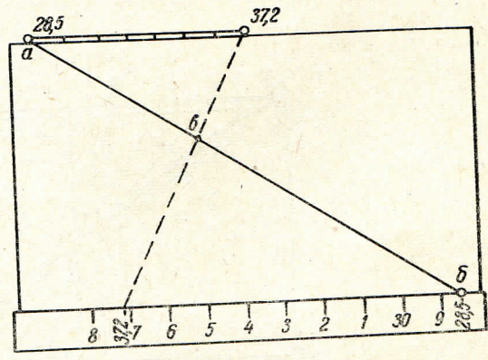
Рис. 5. Шаблон для интерполирования горизонталей.
