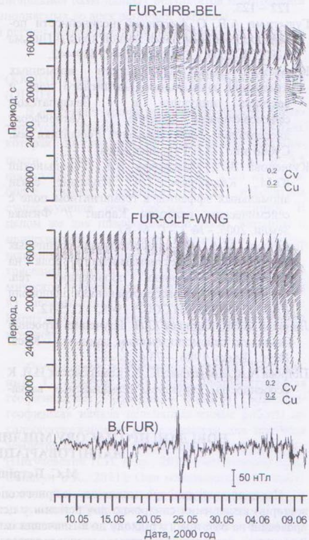
Рис. 2. Спектрально-временное распределение индукционных векторов для двух групп обсерваторий Европейского региона.
