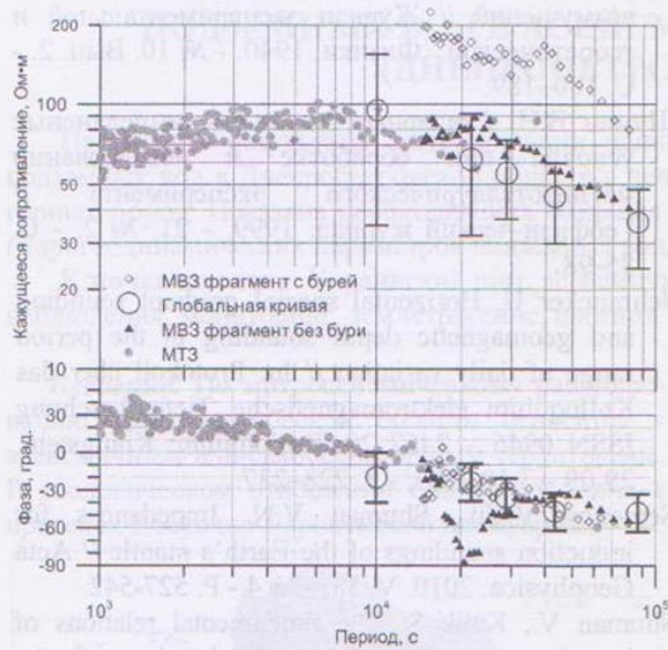
Рис. 1. Совмещенная кривая MT и MB зондирований для обсерватории BEL. Смещение оценок модуля сопротивления MB3 во время магнитной бури.
