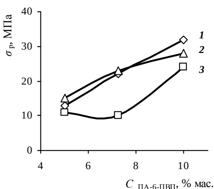
Рис. 4. Залежність руйнівного напруження (а) та відносного видовження (б) за розриву плівок на основі ПА-6/ПВП від концентрації ( C_{\text{ПА-6/ПВП}} ). ПА-6/ПВП=98:2 % мас.; C_{\text{HCOOH}} =84% мас.; T_{\text{уп}} =80 °C. Плівки: 1 – не оброблені; 2 – гідротермооброблені (95 °C); 3 – термооброблені (120 °C) на повітрі
