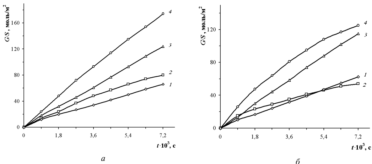
Рис. 8. Кінетичні залежності осмотичної соленепроникності композиційних гідрогелевих мембран (G/S) для NaCl від концентрації модифікованого розчину. Склад гідрогелю: ГЕМА:ПВП:Н 2 О, % мас.: а – 48:12:40, б – 42:18:40; ПА-6:ПВП=95:5 % мас.; С ПА-6/ПВП , % мас.: 1 × 0; 2 × 3; 3 × 5; 4 × 7
