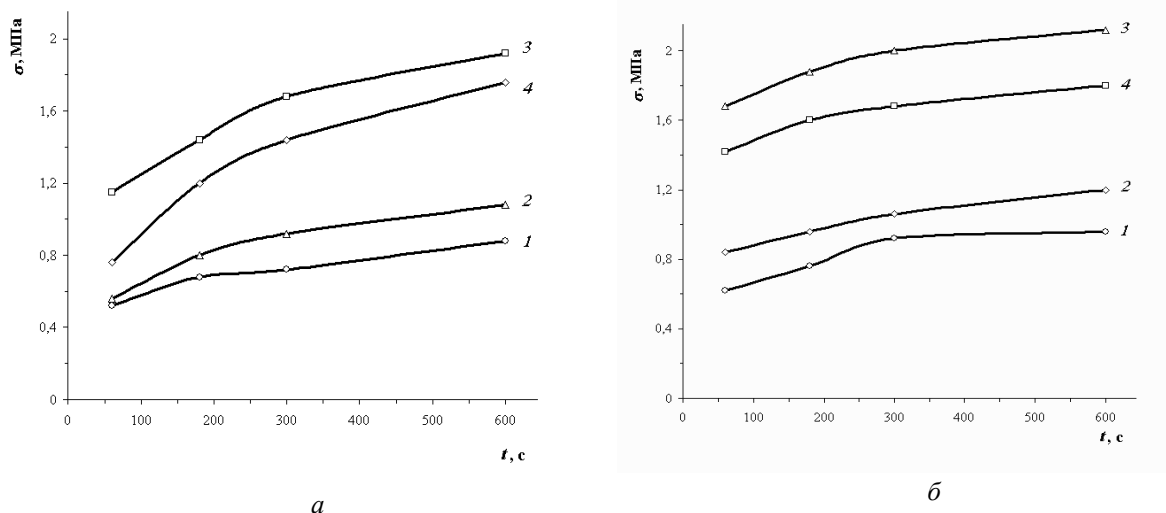
Рис. 7. Залежність міцності композиційних мембран від часу контакту гідрогелю з модифікованим розчином та його концентрацією.
