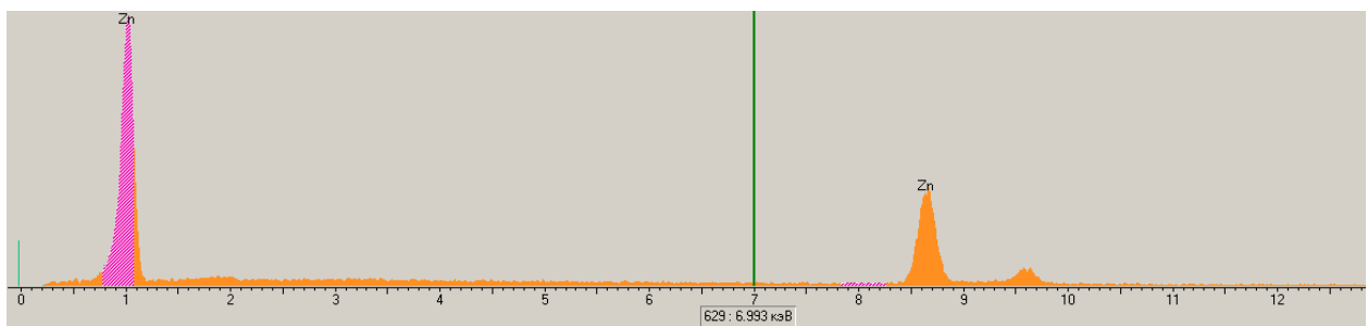
Рис. 4. Спектр характеристичного рентгенівського випромінювання області поверхні, що відповідає найвищому атомному номеру суспензійного полівінілхлориду, одержаної після обробки у кульовому млині в присутності 5 г порошку цинку
