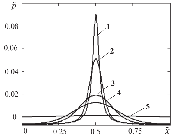
Рис. 2. Розподіл тиску \tilde{p} у шарі при k = 5 \cdot 10^{-13} \text{ м}^2
