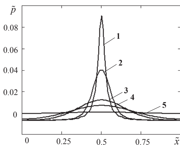
Рис. 7. Розподіл тиску \tilde{p} у шарі при \bar{p} = 100 \cdot 98066,5 Па
