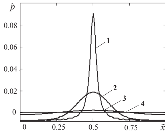
Рис. 3. Розподіл тиску \tilde{p} в шарі при k = 5 \cdot 10^{-12} \text{ м}^2
