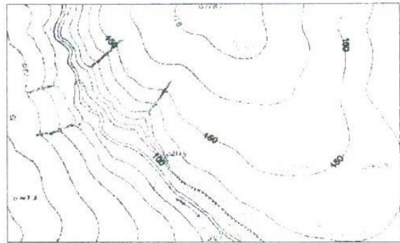
Рис. 2а. ЦМР у вигляді ізоліній типу рідке долиinne розчленування, що не охопило вододіли (III клас)
