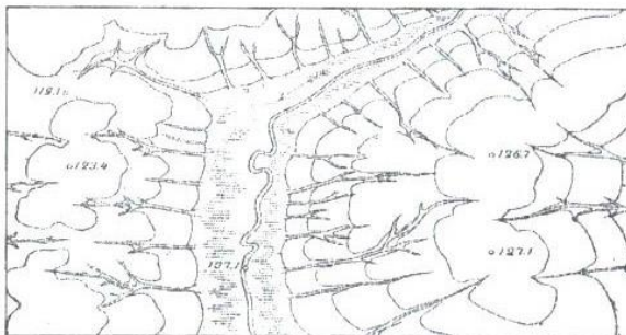
Рис. 5. Долинно-яровий і балково-яровий тип рельєфу, що охопив вододіли (II клас)
