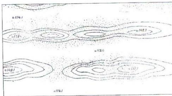
Рис. 10. Рідкогрядовий тип рельєфу (III клас)
