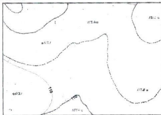
Рис. 1а. ЦМР у вигляді ізоліній типу плоскої нерозчленованої рівнини
