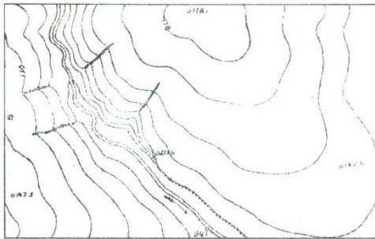
Рис. 2. Тип рідке долиinne розчленування, що не охопило вододіли (III клас)
