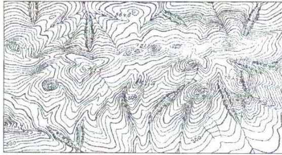
Рис.15. Тип рельєфу середньовисотні гори з різкими формами
