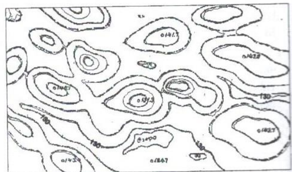
Рис. 9б. ЦМР Частогорбистого типу рельєфу (II клас)
