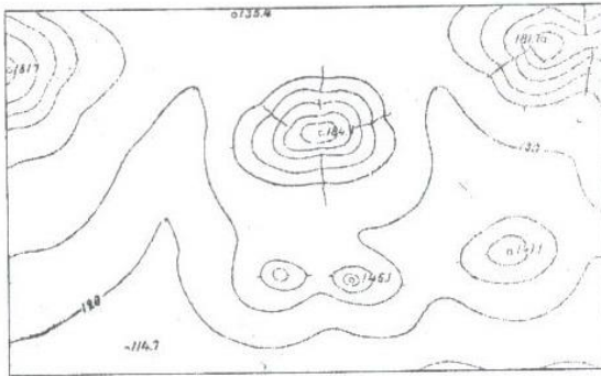
Рис. 8. Рідкогорбистий тип рельєфу (III клас)
