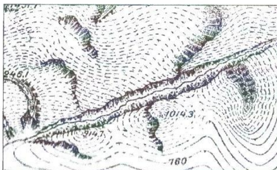
Рис.16. Тип рельєфу середньовисотні гори з альпійськими формами
