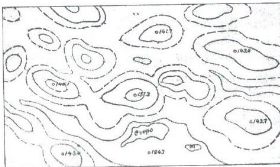
Рис. 9а. Частогорбистий тип рельєфу (II клас)
