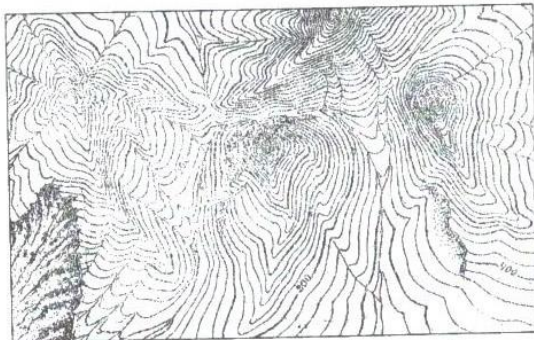
Рис. 13. Тип рельєфу низькі гори з різкими формами
