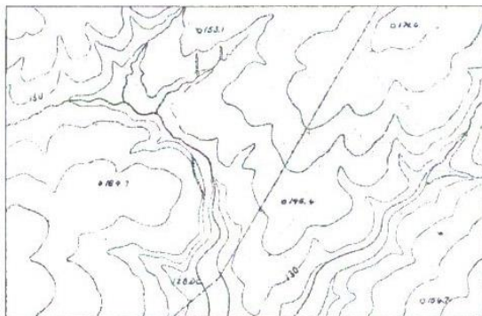
Рис. 3. Тип густе долиinne розчленування, що охопило вододіли (II клас)
