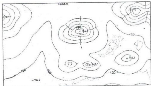
Рис. 8а. ЦМР рідкогорбистого типу рельєфу (III клас)
