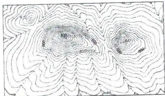
Рис.14а. ЦМР типу середньовисотні гори з м'якими формами
