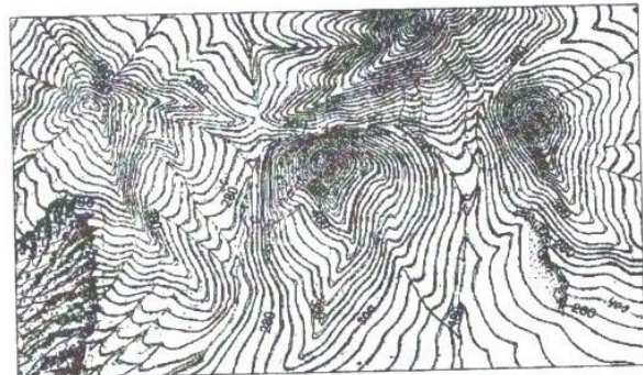
Рис. 13а. ЦМР типу низькі гори з різкими формами рельєфу
