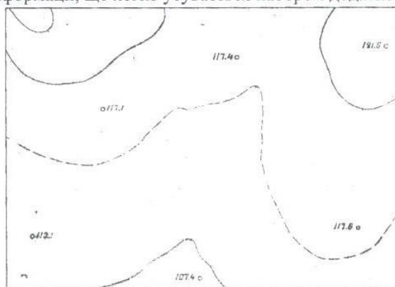
Рис. 1. Тип рельєфу плоска нерозчленована рівнина
