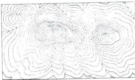
Рис.14. Тип рельєфу середньовисотні гори з м'якими формами
