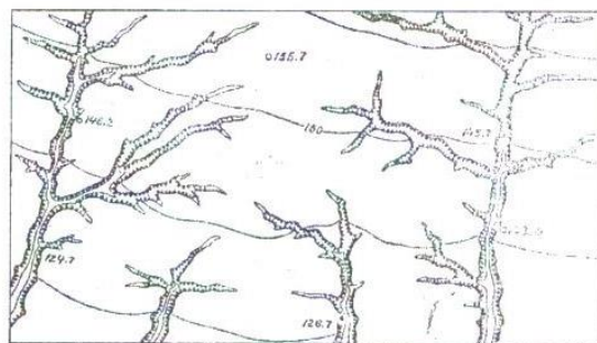
Рис.7. Яровий тип рельєфу з високорозвиненою мережею (III клас)
