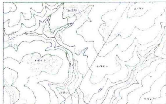
Рис. 3а. ЦМР типу густе долиinne розчленування, що охопило вододіли (II клас)
