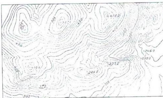
Рис. 12. Тип рельєфу низькі гори з м'якими формами
