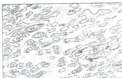
Рис. 11а. ЦМР частогрядового типу рельєфу
