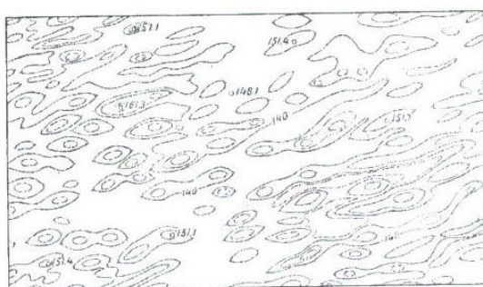
Рис. 11. Частогрядовий тип рельєфу
