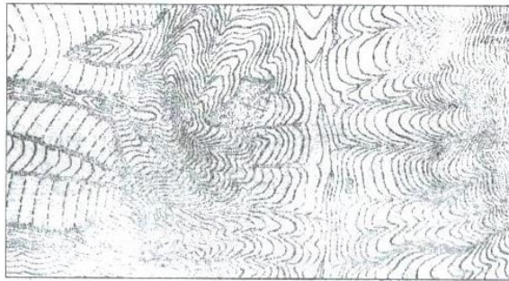
Рис.17. Тип рельєфу гори з різким альпійським розчленуванням
