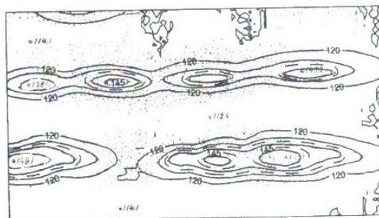
Рис. 10а. ЦМР рідкогрядового типу рельєфу (III клас)
