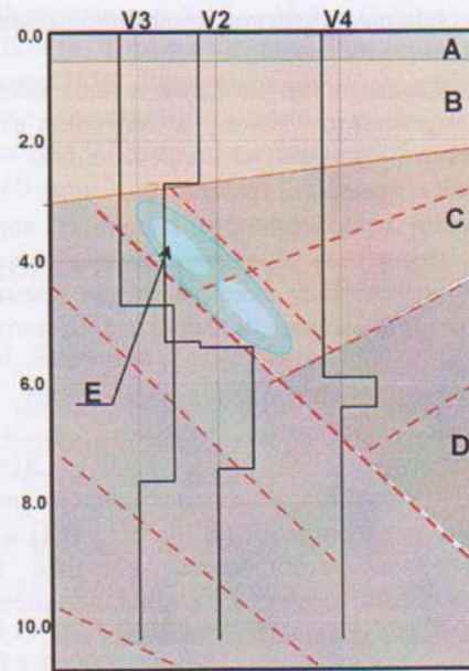
Рис. 4. Геолого-геофизический разрез зоны фильтрационного водного потока по профилю № 3.
