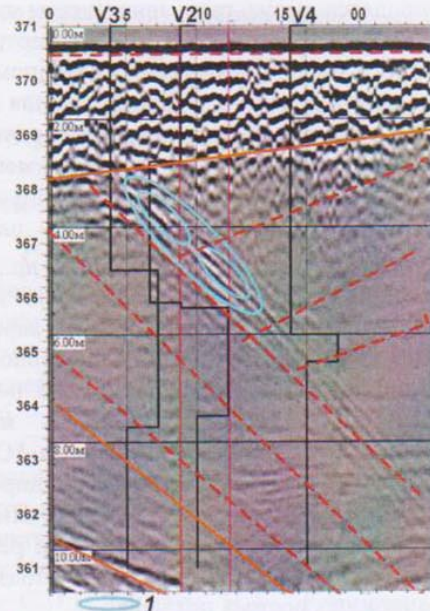
Рис. 3. Георадарный разрез зоны фильтрационного водного потока по профилю № 3. 1 – зона водного потока
