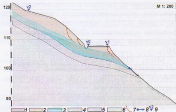
Рис. 2. Поперечный разрез оползневой зоны.
