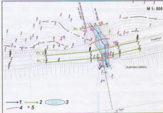
Рис. 1. Карта зоны подземного водного потока на оползневом участке дороги.
