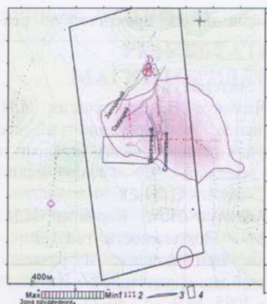
Рис. 1. Карта аномалий типа "зона уранового оруденения" на площади работ.
