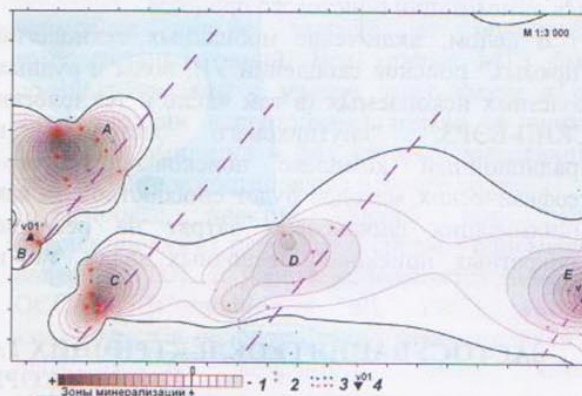
Рис. 4. Карта аномалий типа "зона платинорудного оруденения" на участке "АР" (по данным съемки СКИП).
