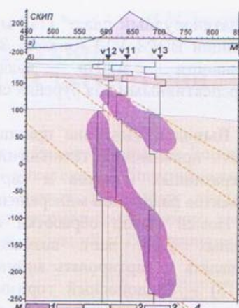
Рис. 3. Вертикальный разрез аномальной зоны типа "урановое оруденение", профиль 1.
