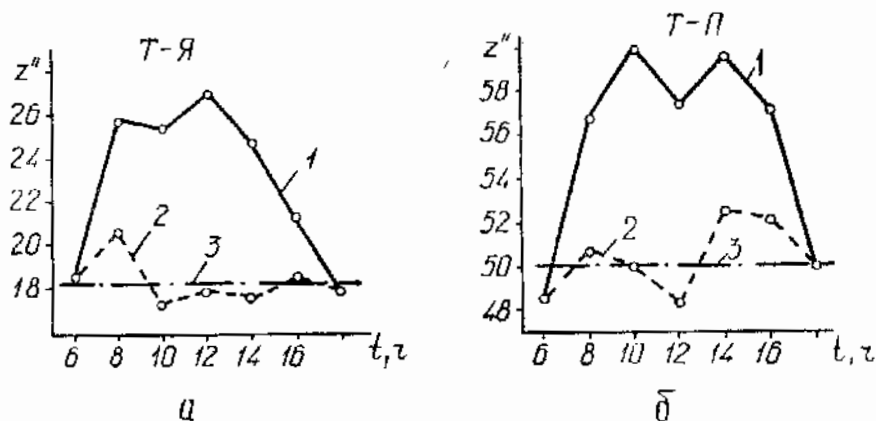
Рис. 2. Графики измеренных и редуцированных зенитных расстояний по линиям Т-Я (а) и Т-П (б):
