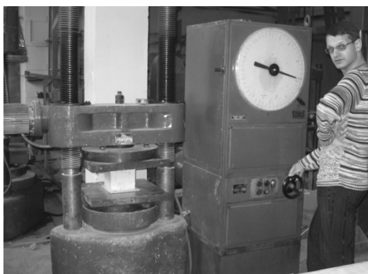
Рис. 4. Процес випробування еталонних взірців-кубів на стиск та загальний вигляд випробуваного взірця
