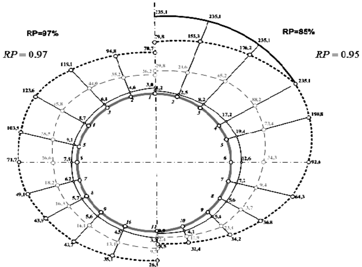
Рис. 2. Розподіл напружень у металевій гофрованій конструкції
