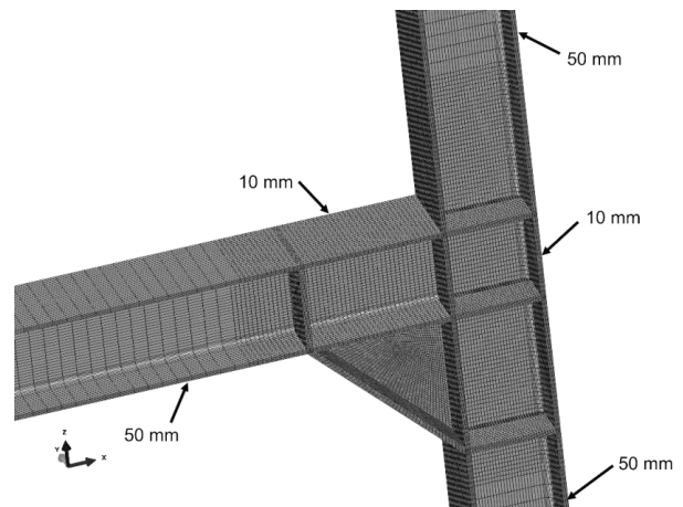
Fig. 6. Mesh – frame
