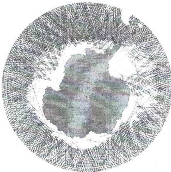
Рис. 1. Розподіл вихідної альтиметричної інформації на регіон Антарктики
