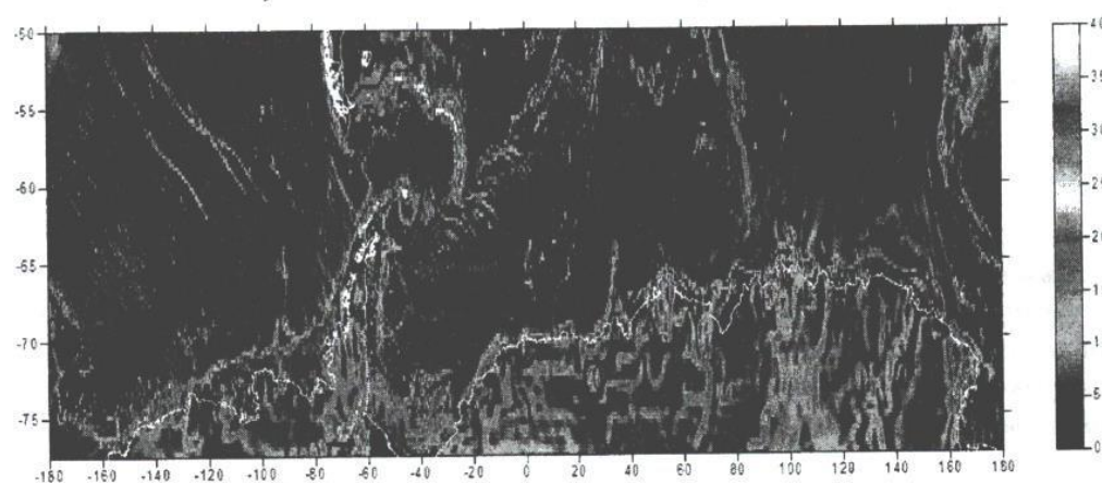
Рис. 5. Побудоване поле складових відхилень прямовисної лінії \theta на регіон Антарктики
