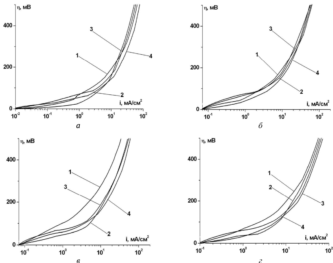
Рис. 2. Перенапруга катодних процесів за наявності сульфідної плівки на поверхні феритно-перлітної (а), сорбітної (б), трооститної (в) і мартенситної (г) структури сталі 45 у розчині 0,5 % CH_3COOH + 5 % NaCl : 1 – Ст.45; 2 – Ст.45 – FeS_2 ; 3 – Ст.45 – FeS ; 4 – Ст.45 – Fe_9S_8
