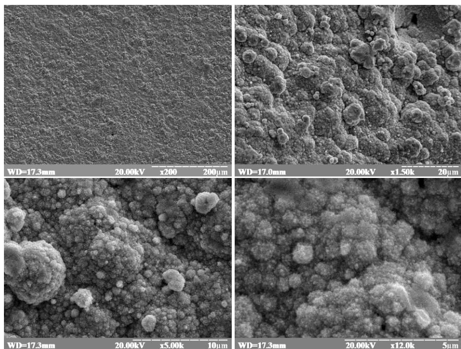
Рис. 6. Мікрофотографії поверхні мідненого ПВХ пластикату
