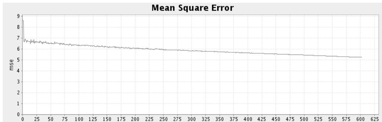
Рис. 14. Графік зміни MSE упродовж навчання кожні 100 ітерацій
