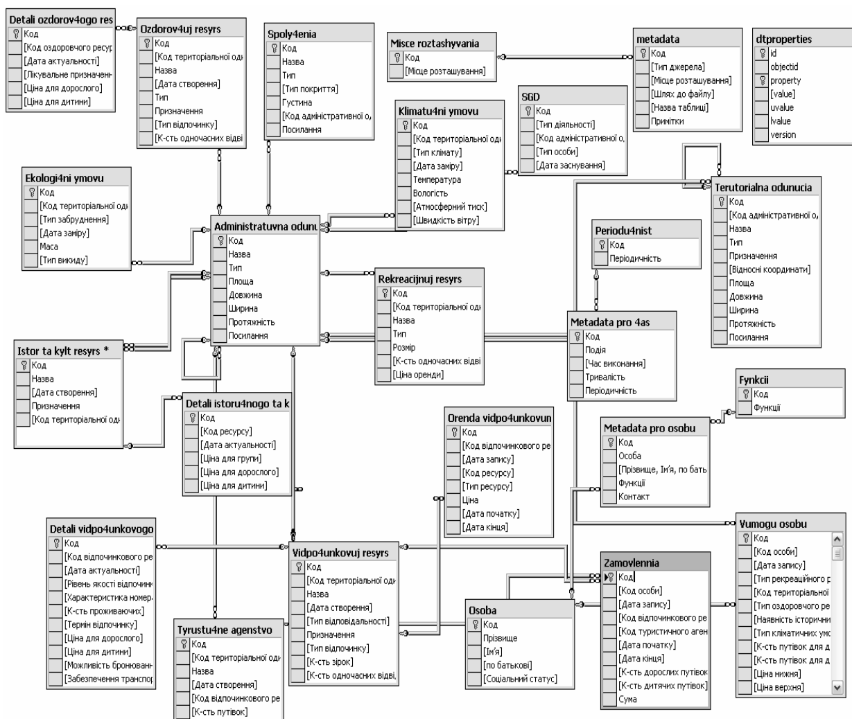
Рис. 5. Схема серверної бази даних
