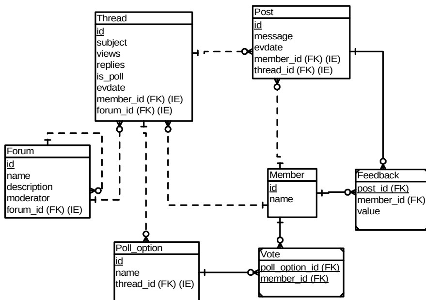
Рис. 3. Інформаційна модель Веб-форуму
