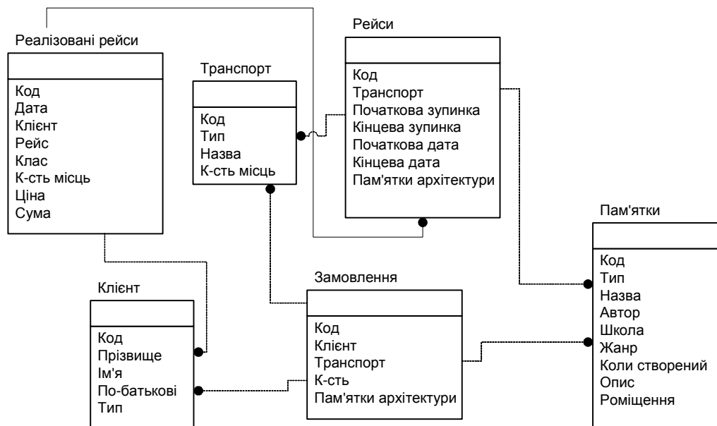
Рис. 7. Можлива логічна модель даних туристичного агентства
