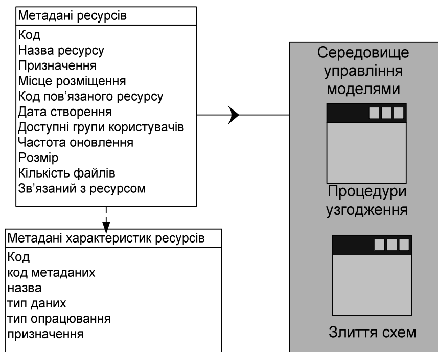
Рис. 3. Схема каталогу простору даних
