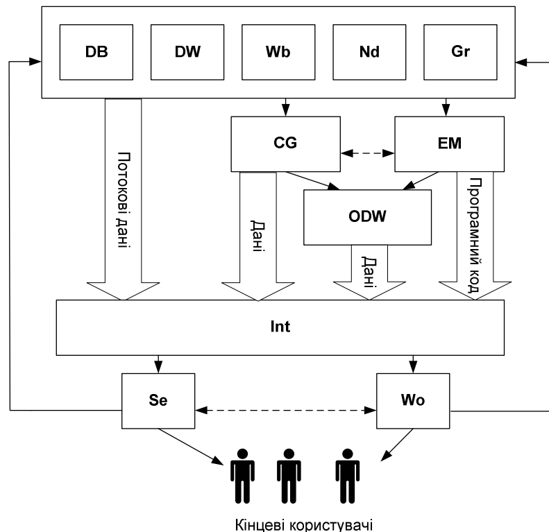
Рис. 4. Схema зв'язку між елементами сховища даних
