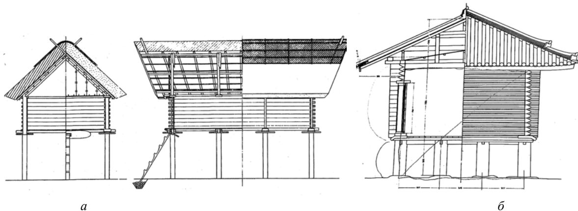
Рис. 1. Японські зерносховища “такаюка” змішаної зрубно-каркасної конструкції, відновлене поселення Торо, префектура Шідзуока, Бронза (а); зрубний релікварій храму Тошьюдайджі, Нара, VIII ст. (обмірні креслення реставраційної майстерні Т. Сакураї, за участю автора) (б)
