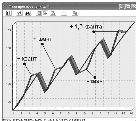
Рис. 5. Результати нейроматематичного моделювання НЕМ з чотирма входами (похибки квантування в тестовій вибірці входів): а, б – значення напруги на шині ПС5 (тестування) НЕМ
