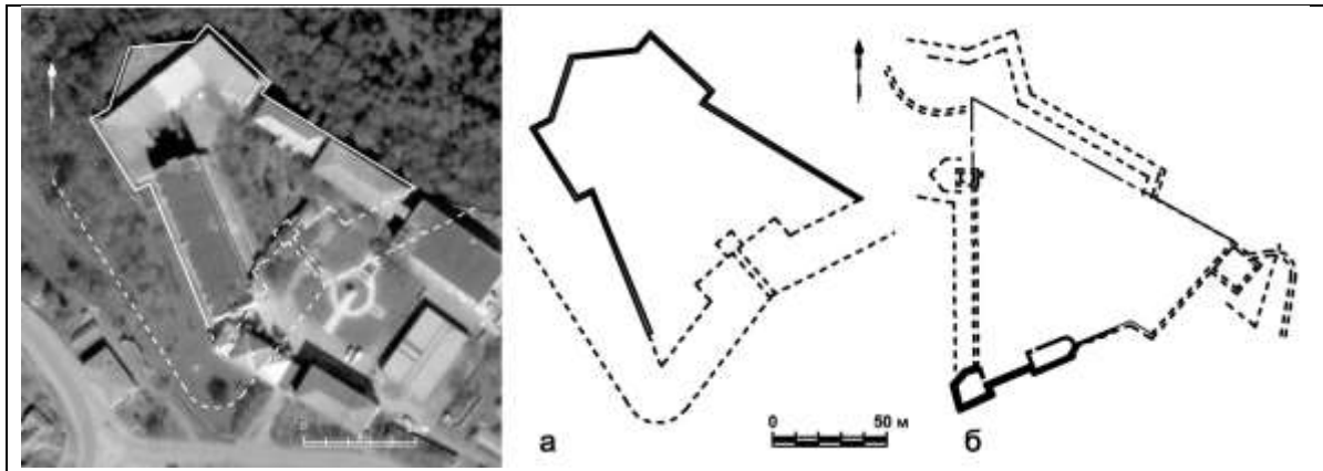
Рис. 12. а) Схема замку у Ягільниці (креслення автора) накладена на знімок з супутника (Google maps, 2020). б) Схема замку у Галичі, прорис автора з плану 1795р. опублікованого у праці Л. Поліщук (Поліщук, 2011, с. 98-104)
