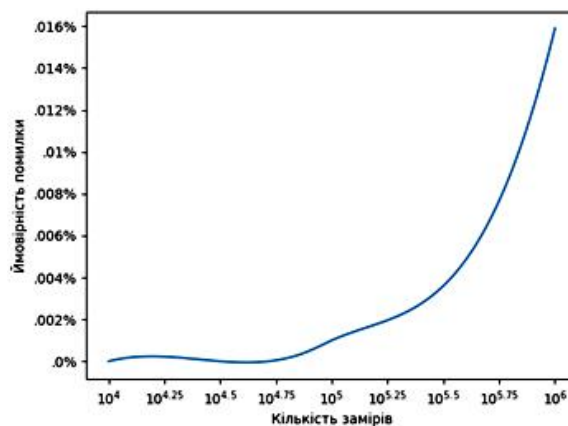
Рис. 13. Залежність ймовірності помилки від кількості замірів
