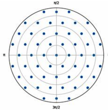
Рис. 3. Сигнальне сузір'я 55-АМБС
