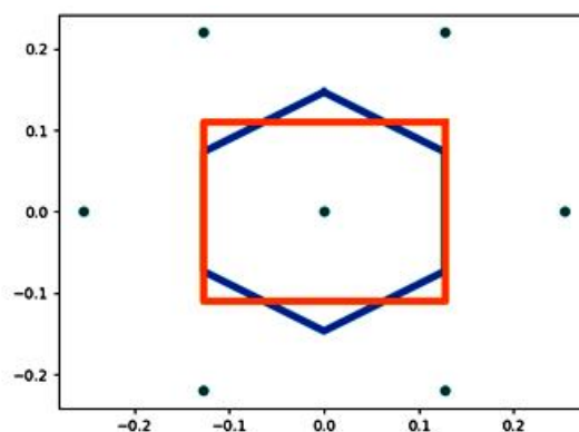
Рис. 5. Порівняння порогової комірки із коміркою Вороного
