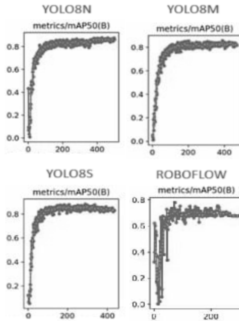
Рис. 3. Метрики нейронних мереж YOLOv8S моделей.
