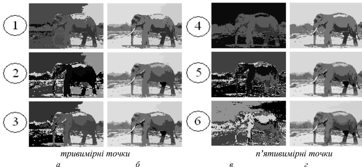
Рис. 8. Результати декомпозиції простору та каскадного згортання: 1 – l = (2, 2, 2) ; 2 – l = (3, 3, 3) ; 3 – l = (4, 4, 4) ; 4 – l = (2, 2, 2, 2, 2) ; 5 – l = (2, 2, 4, 4, 4) ; 6 – l = (1, 1, 9, 9, 9) ; а, в – кластери, розфарбовані випадковим кольором; б, г – кластери, розфарбовані їх зваженою яскравістю
