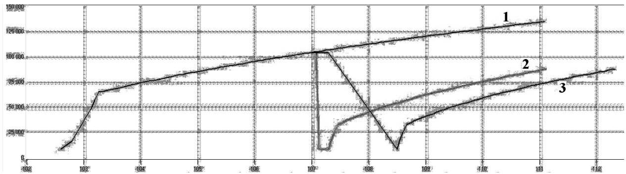
Рис. 2. Змінення CWND: лінія 1 – Повільний старт і Уникнення перевантаження; лінія 2 – Tahoe за однієї втрати сегмента; лінія 3 – Reno за однієї втрати сегмента
