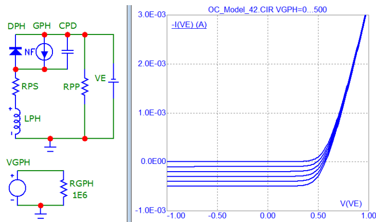
Рис. 9. Схема BAX фоточутливого модуля S\_PHD для масиву значень фотоструму I(GPH) = I(VGPH)
