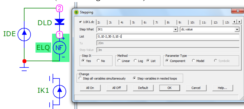
Рис. 6. Приклад специфікації для методу дослідження типу Stepping
