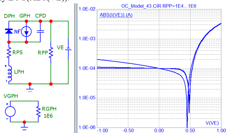
Рис. 10. BAX фоточутливого компоненту S\_PHD для масиву значень опору RPP в логарифмічному масштабі
