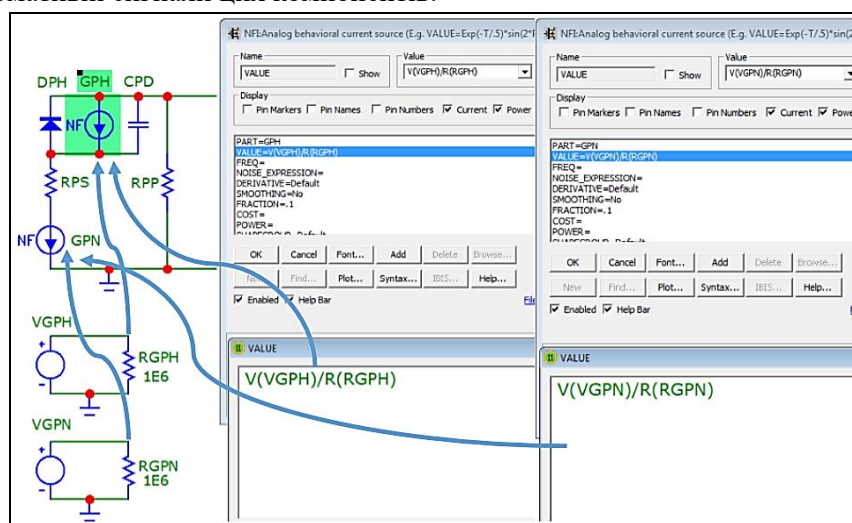
Рис. 8. Схема заміщення з двома керованими джерелами струму
