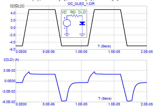
Рис. 4. Процес перемикавання струму в структурі OLED
