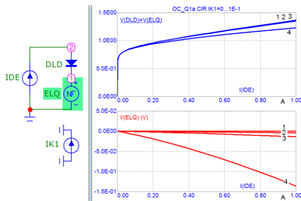
Рис. 7. BAX діода V(DLD) = f(I(IDE)) (зверху) та функціональна залежність напруги джерела ELQ V(ELQ) = f(I(IDE)) (знизу) – метод Stepping
