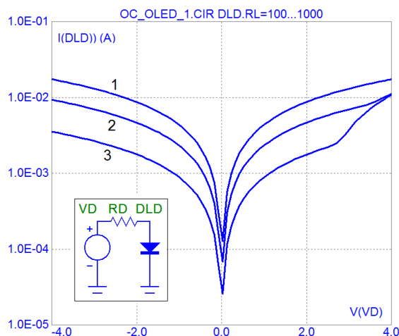
Рис. 3. BAX структури OLED при R_{LP} = 100 \text{ Ом} (1), 300 \text{ Ом} (2), 1000 \text{ Ом} (3)
