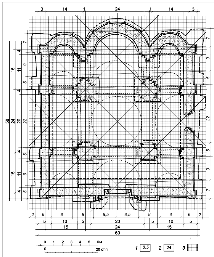
Рис. 8. Метрологічний аналіз плану церкви св. Пантелеймона у мірничих стопах по 30 см: 1 – на рівні підмурків; 2 – на рівні стін; 3 – сітка 30×30 см
