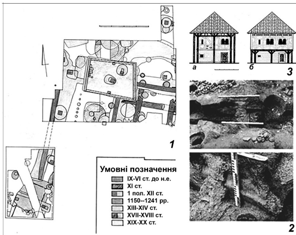
Рис. 3. Палацові споруди першої половини XII ст. під Митрополичими палатами в Крилосі: 1 – плани розкопів; 2 – згорілі сліди фундаментів (фото автора); 3 – варіанти гіпотетичних реконструкцій. (рис. В. Петрика)
