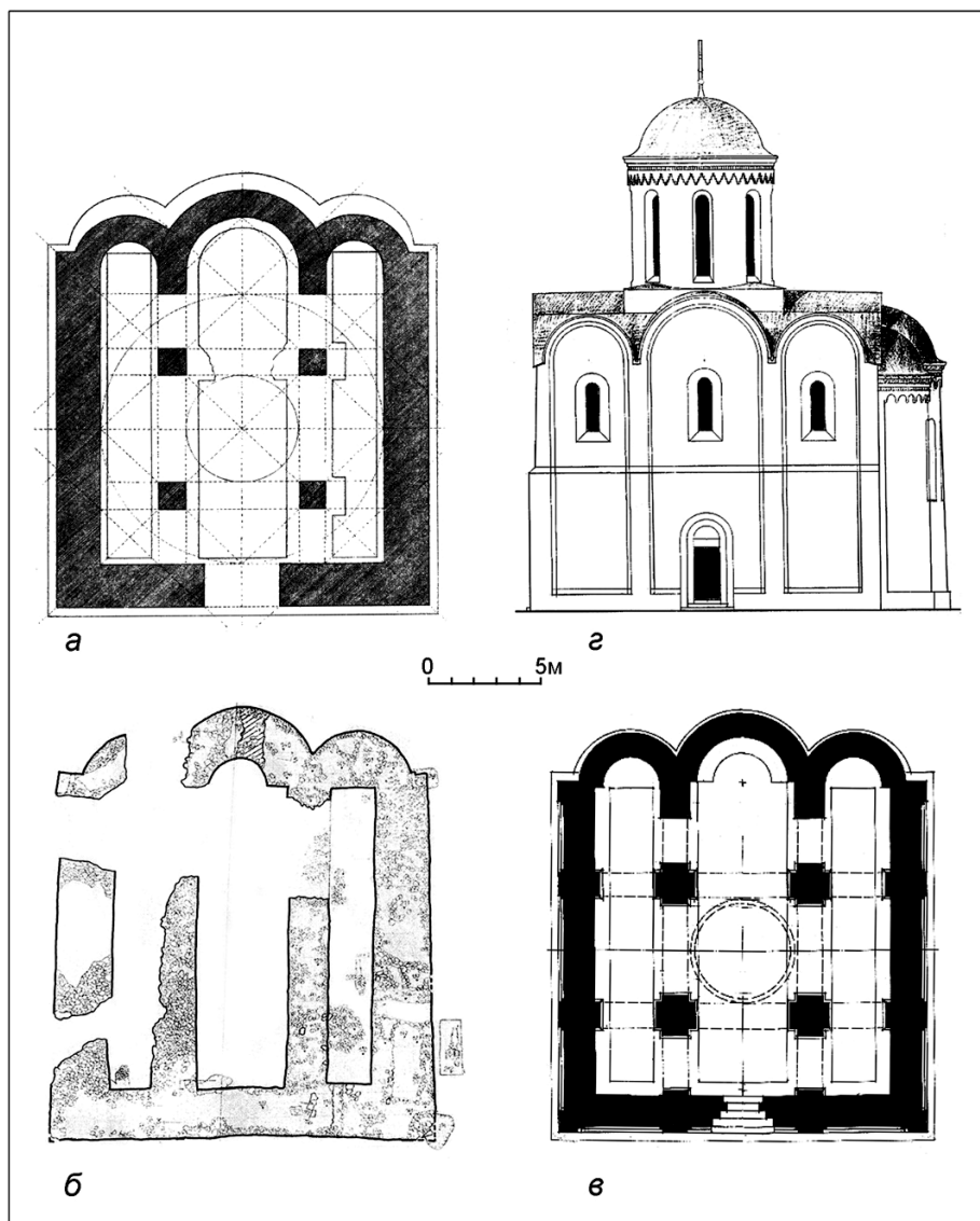
Рис. 5. Церква Спаса на горі Карпиця: а – планувальна реконструкція за Ю. Захарієвичем; б – план підмурків за О. Іоаннісяном; в – реконструкція плану на рівні наземних стін; г – реконструкція південного фасаду церкви (рис. В. Петрика)
