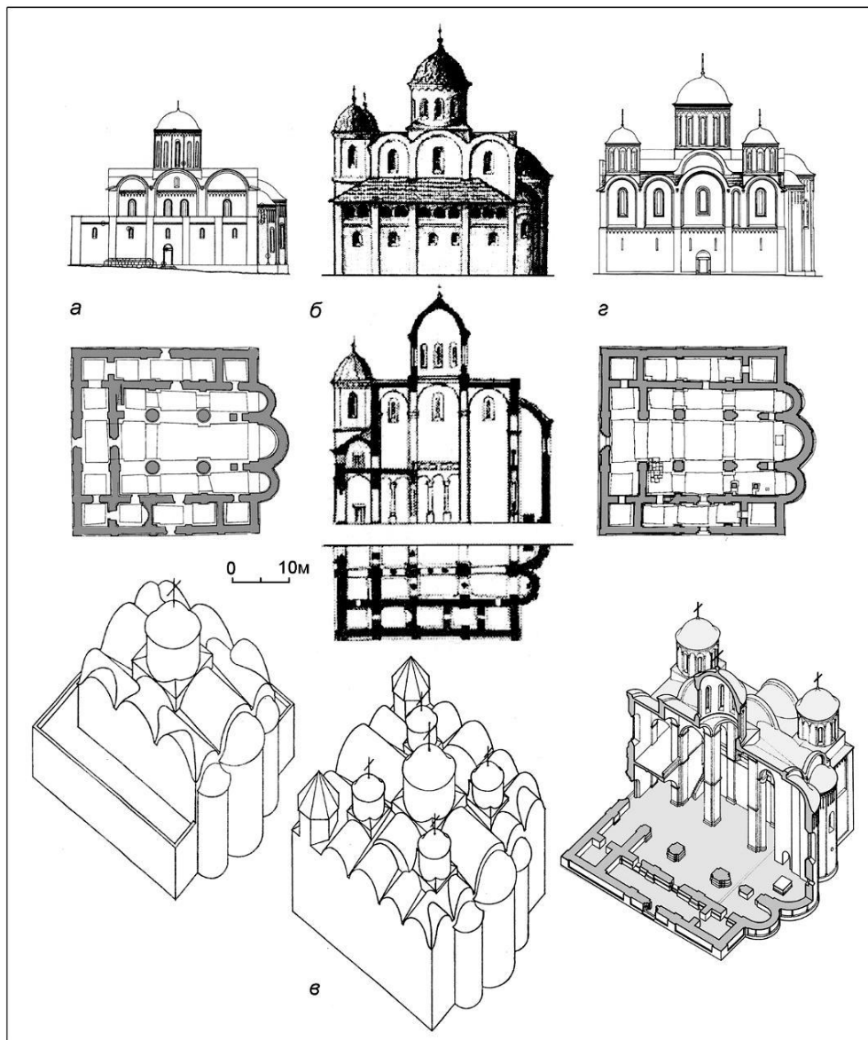
Рис. 6. Графічні реконструкції галицького Успенського собору:
