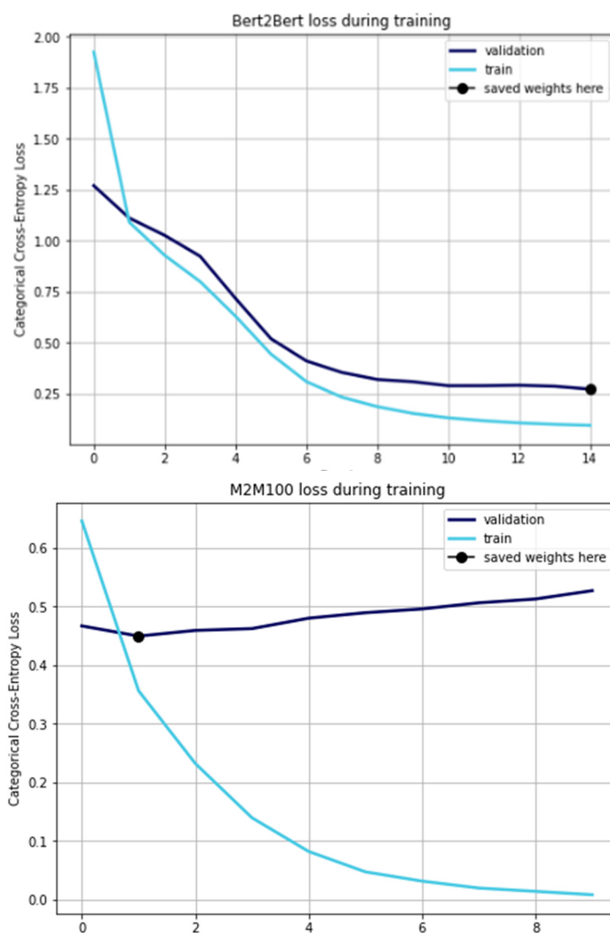
Рис. 22. Крива функції втрат при навчанні та тестуванні нейронної мережі
