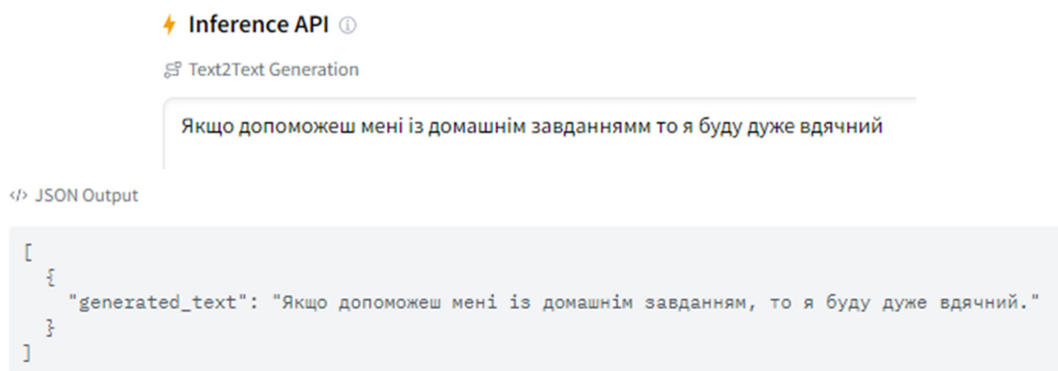
Рис. 7. Приклад виправлення пунктуаційних помилок на основі моделі GEC команди Правописця
